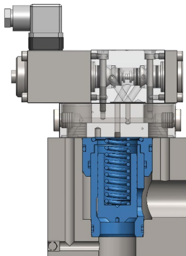
Einbau und Ansteuerung eines Einbauventils
