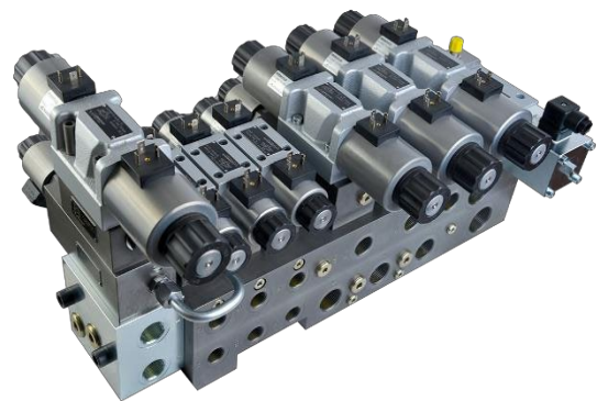
Kundenspezifische Steuereinheit
